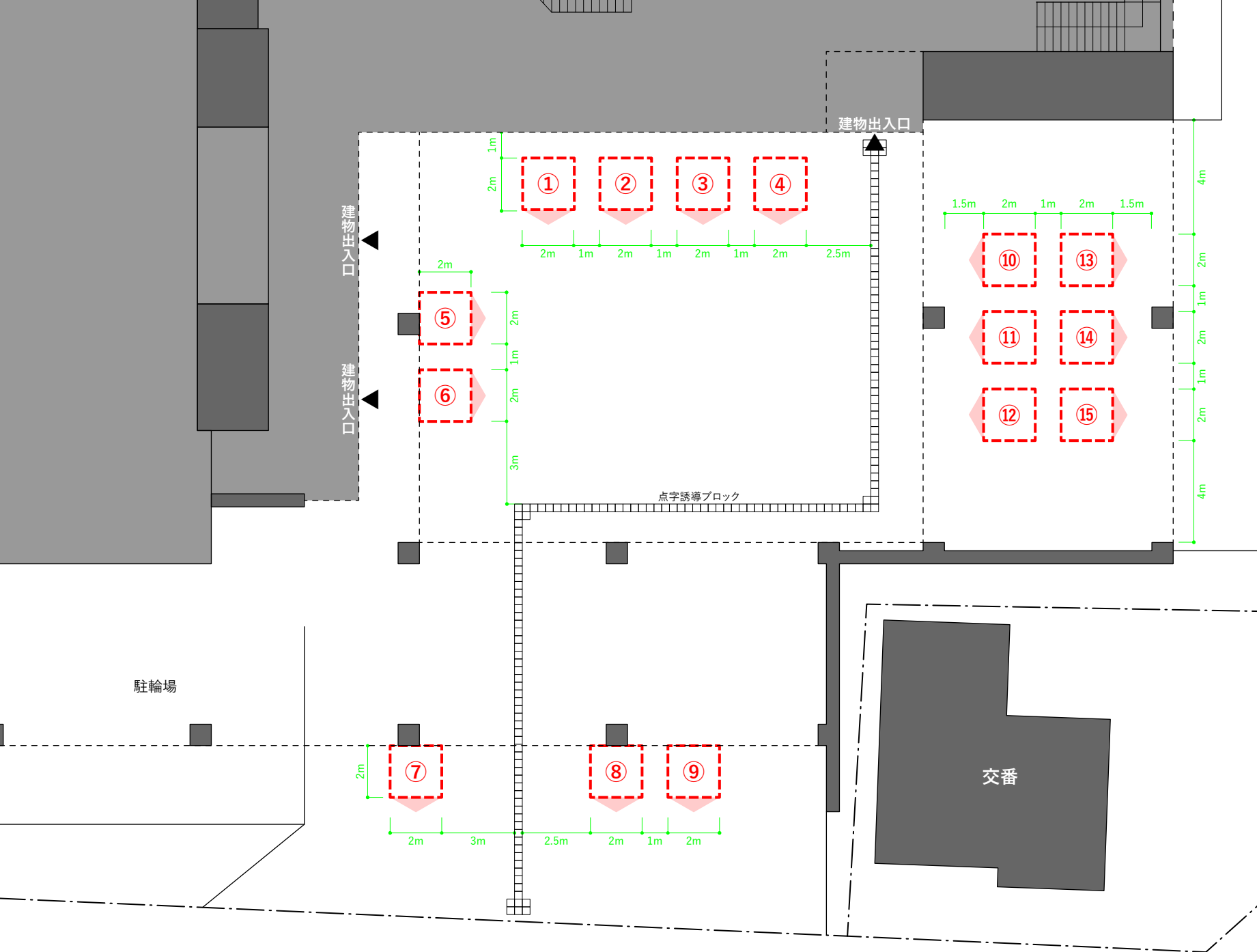
みそのいち出店区画配置図 [B]美園コミュニティセンター交流広場 (A4:1/200)
